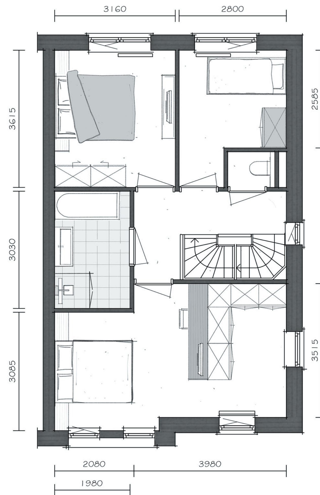
eerste verdieping
