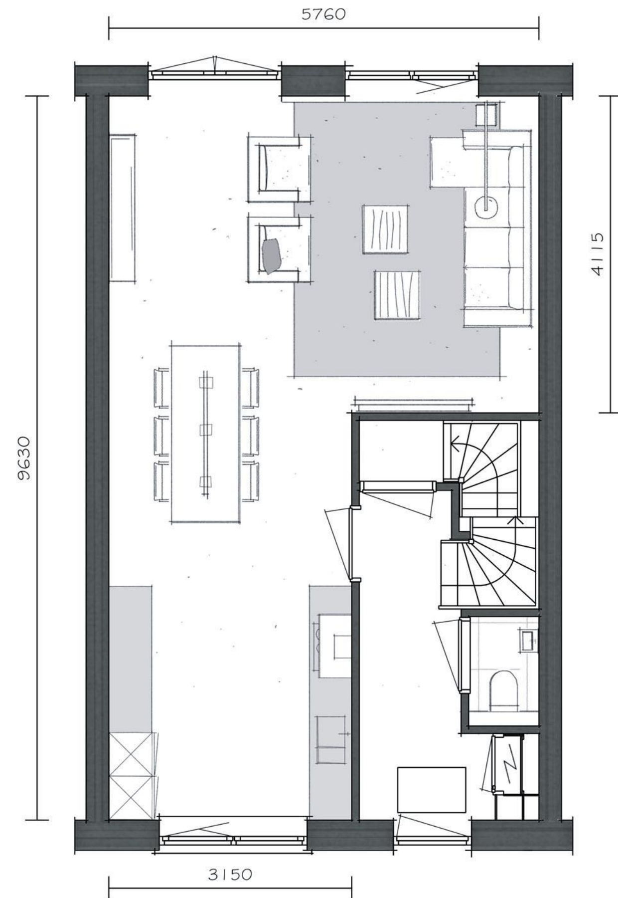
begane grond
