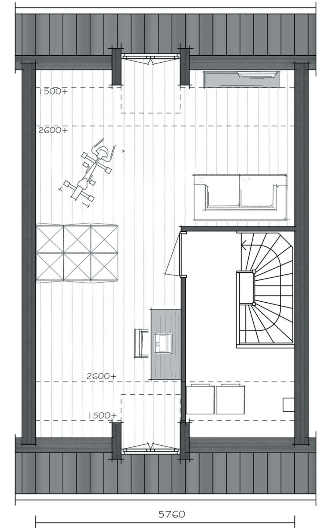
tweede verdieping
