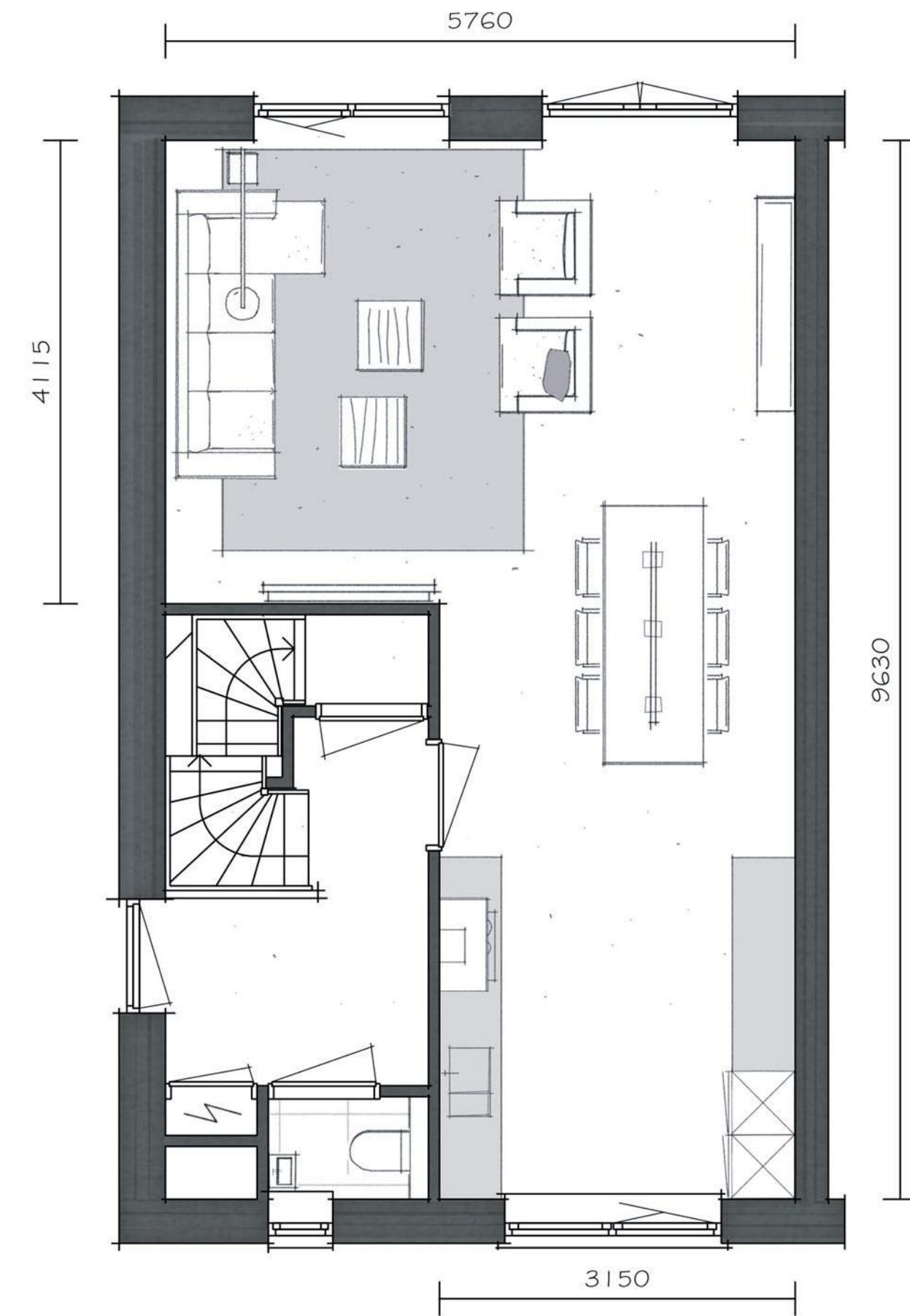
begane grond
