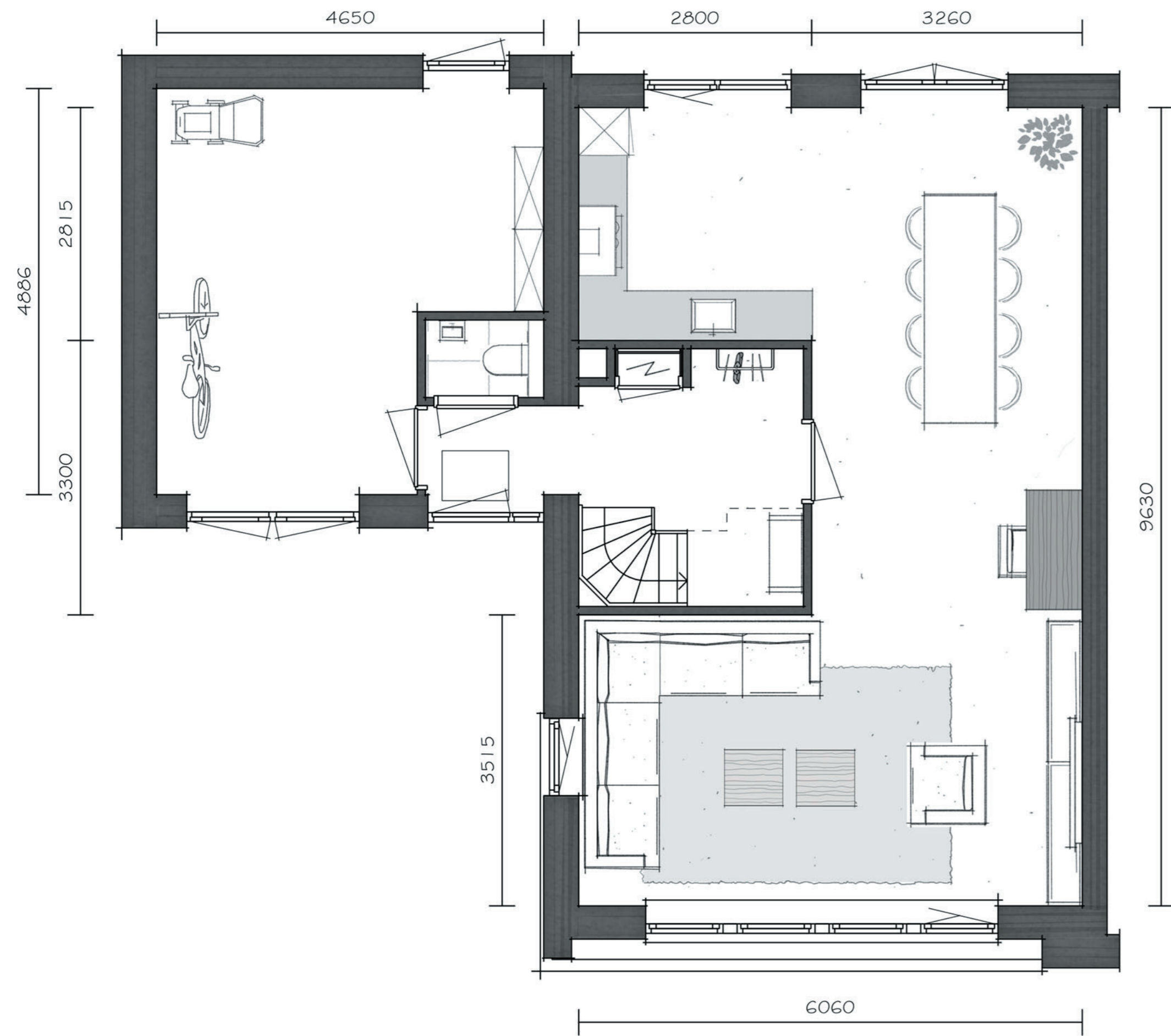
begane grond
