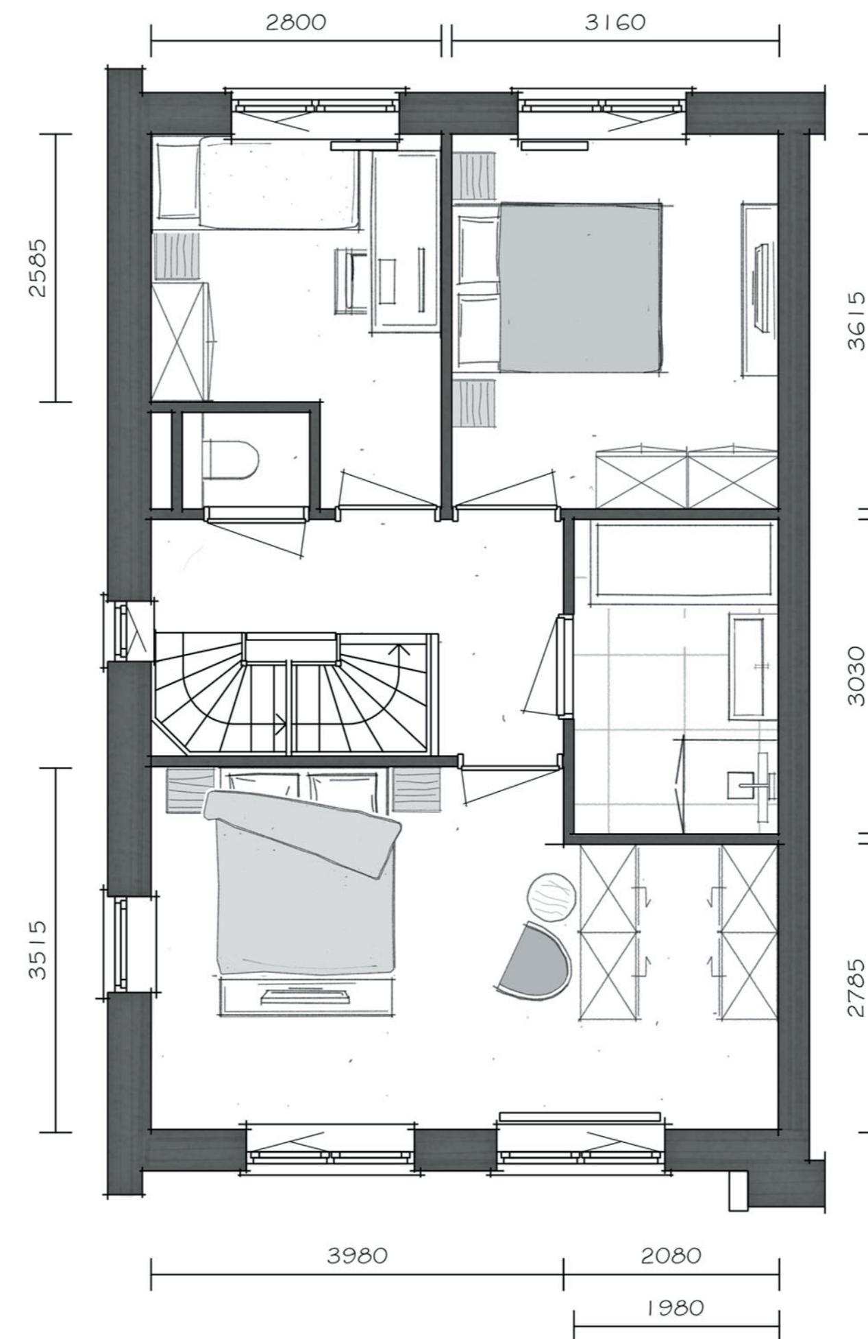
eerste verdieping
