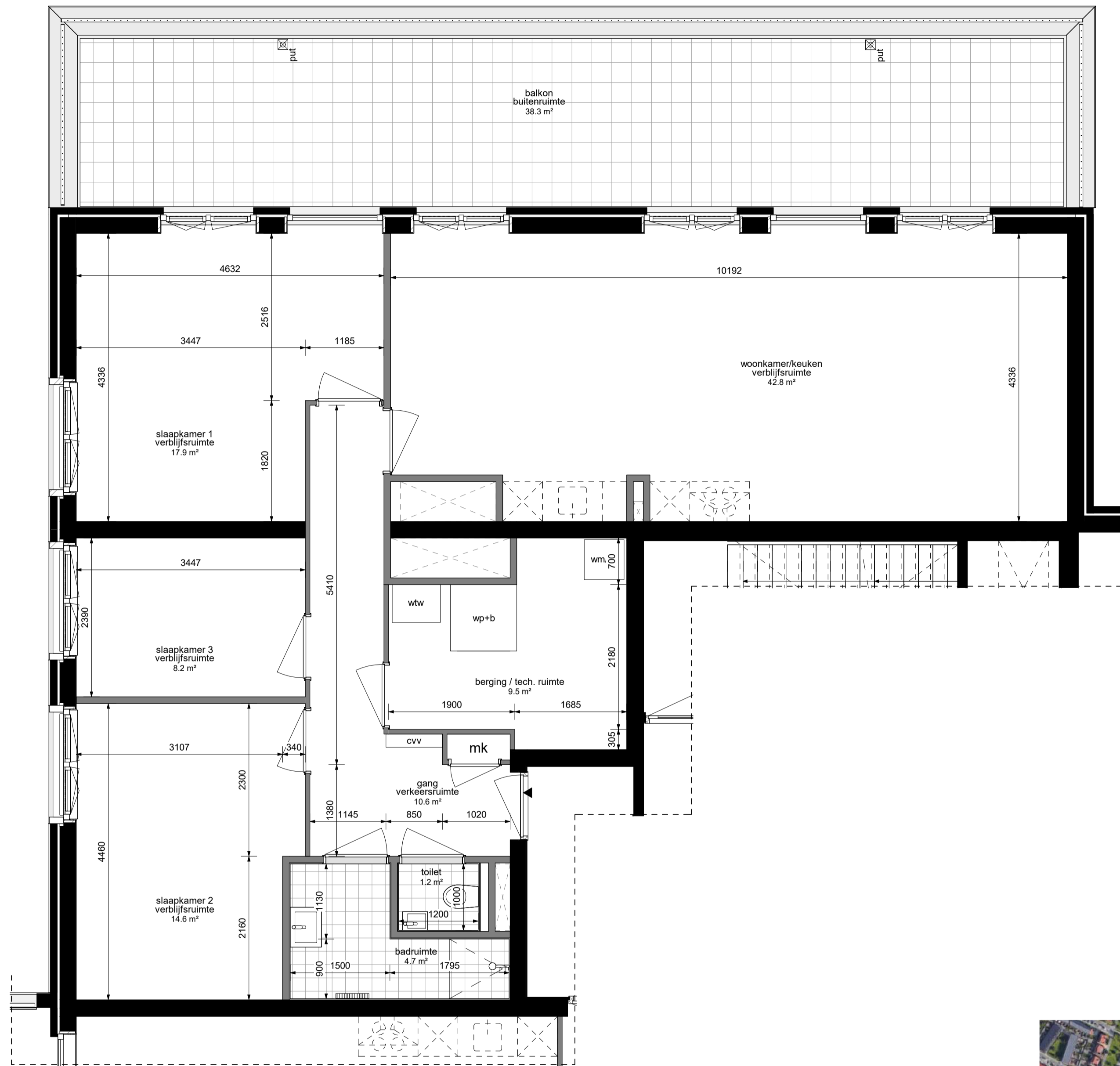
Bouwnummer 91 schaal 1 : 50
