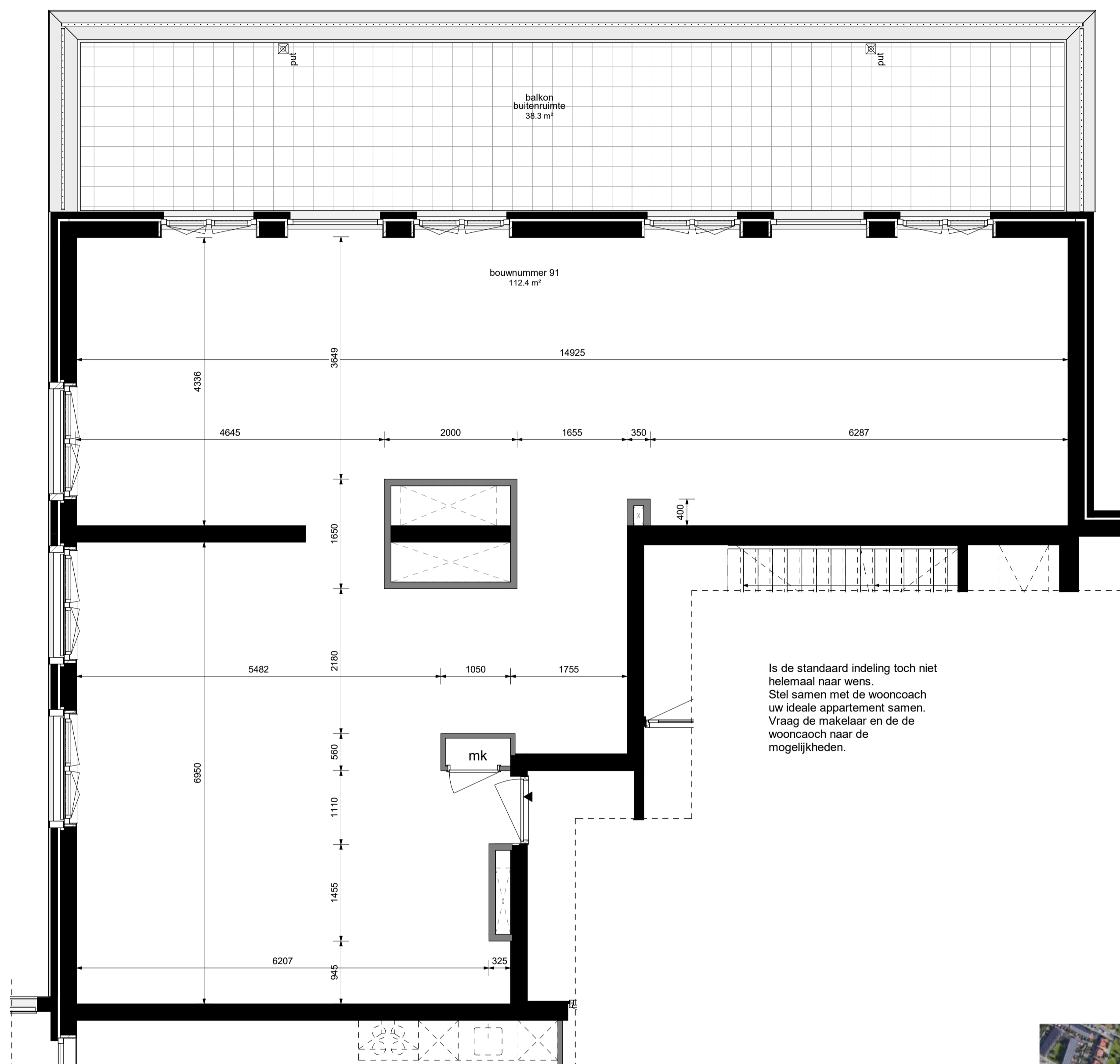
Bouwnummer 91 leeg schaal 1 : 50
