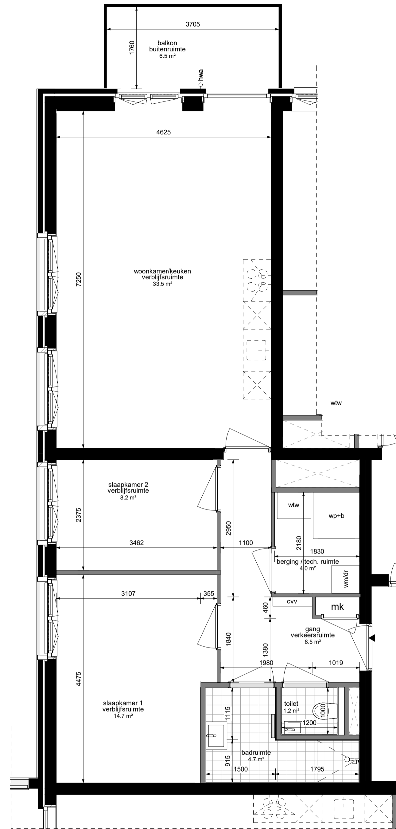
Bouwnummer 80 schaal 1 : 50
