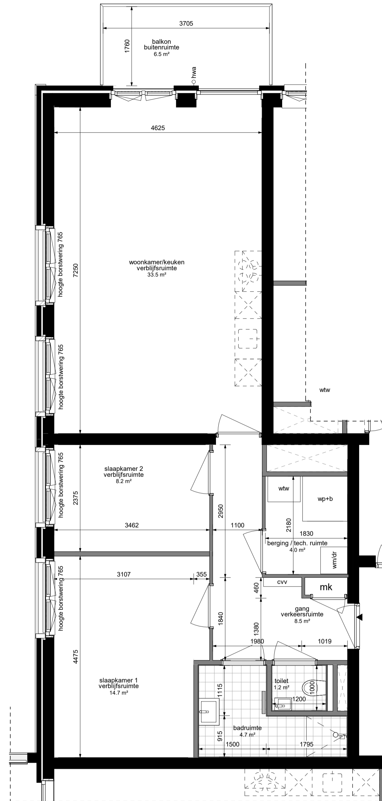
Bouwnummer 48 schaal 1 : 50
